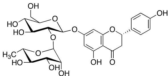
Naringin
