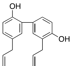
Honokiol
